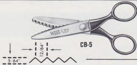
Actual Size Pink 5 1/2" and 7 1/2" Pinkers
